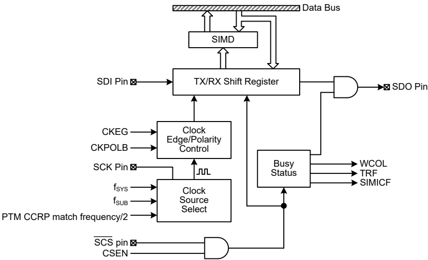
SPI 方框图
