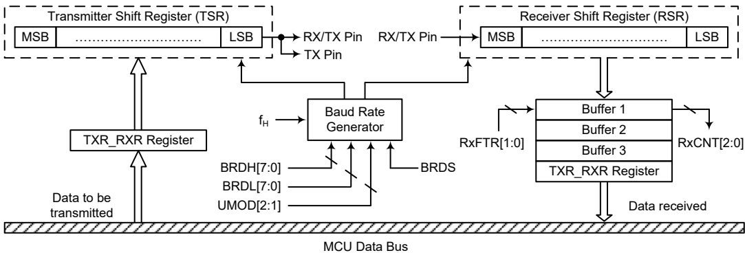
UART 数据传输方框图 – SWM=1
