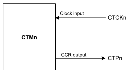
CTM 功能引脚框图 (n=0~1)
