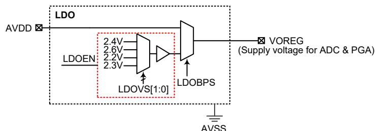
内部电源供电方框图
