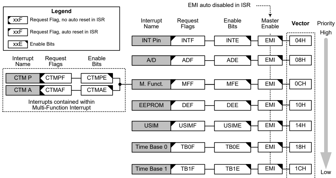
中断结构
