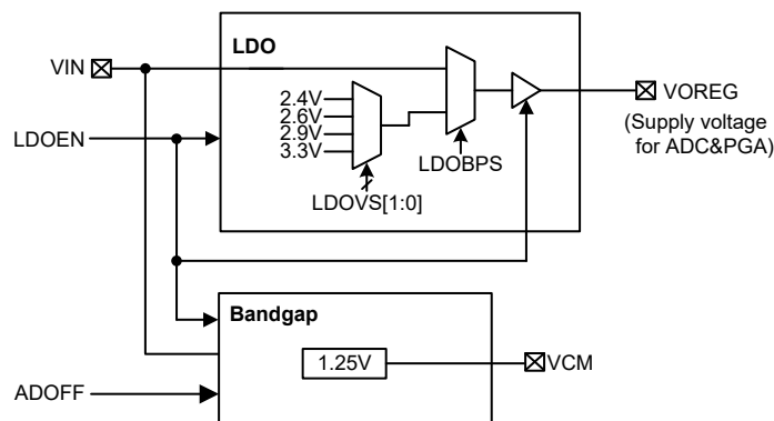
内部电源供电方框图
