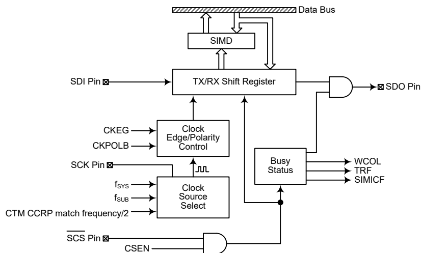
SPI 方框图
