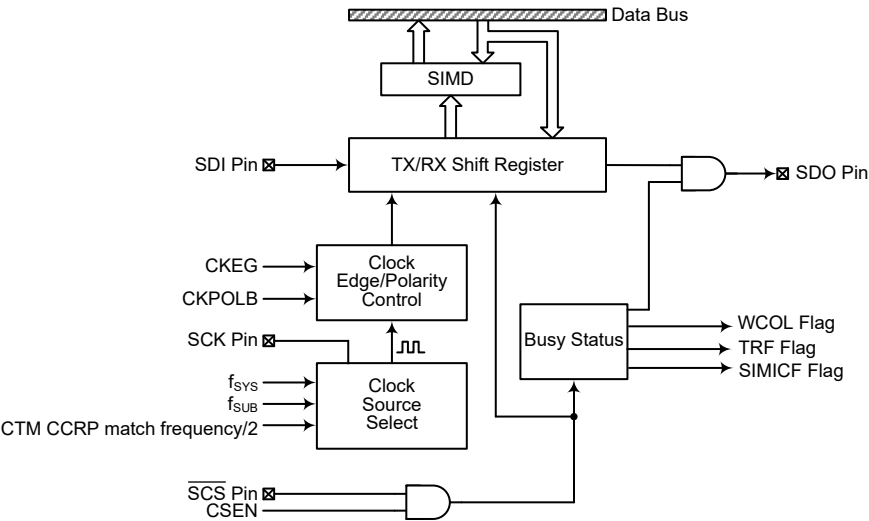
SPI 方框图
