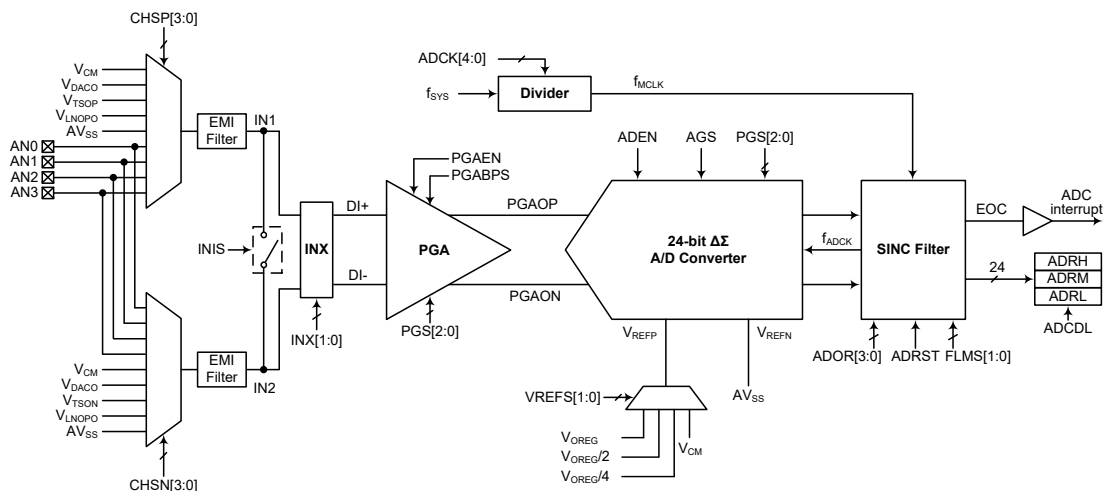
A/D 转换器结构
