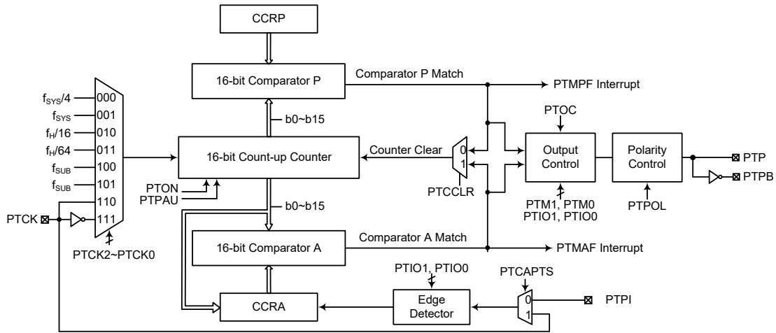
16-bit 周期型 TM 方框图
