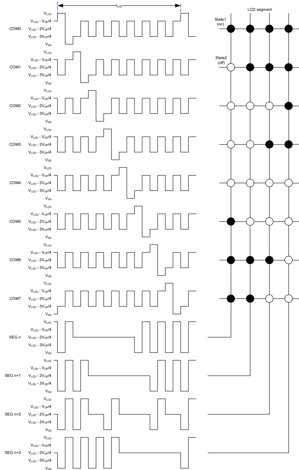
1/8 duty 和 1/4 bias 驱动模式波形图 ( V_{Op}=V_{LCD}-V_{SS} )
