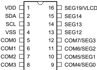
HT16C21A 16 NSOP-A
