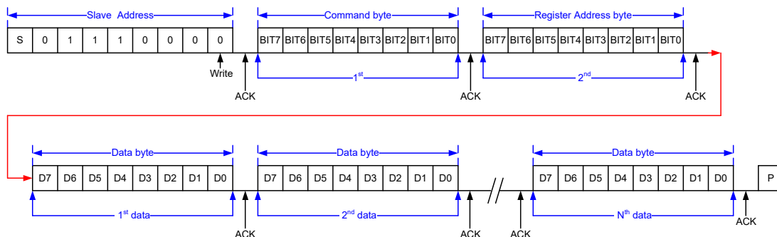
N 字节显示 RAM 数据写入操作
