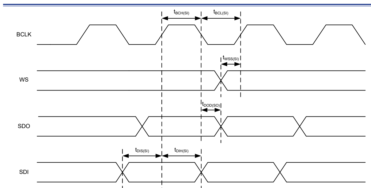
图 9. PS 从机模式时序图
