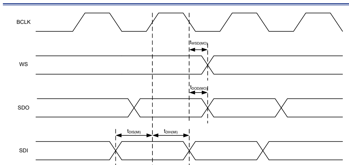
图 8. PS 主机模式时序图
