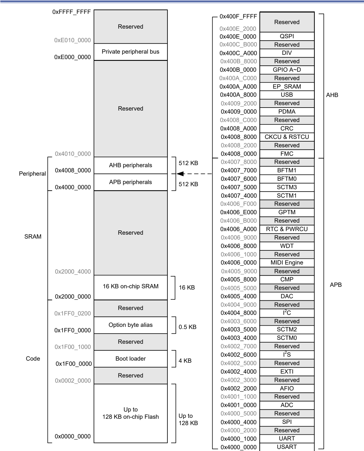
图 2. 存储器映射
