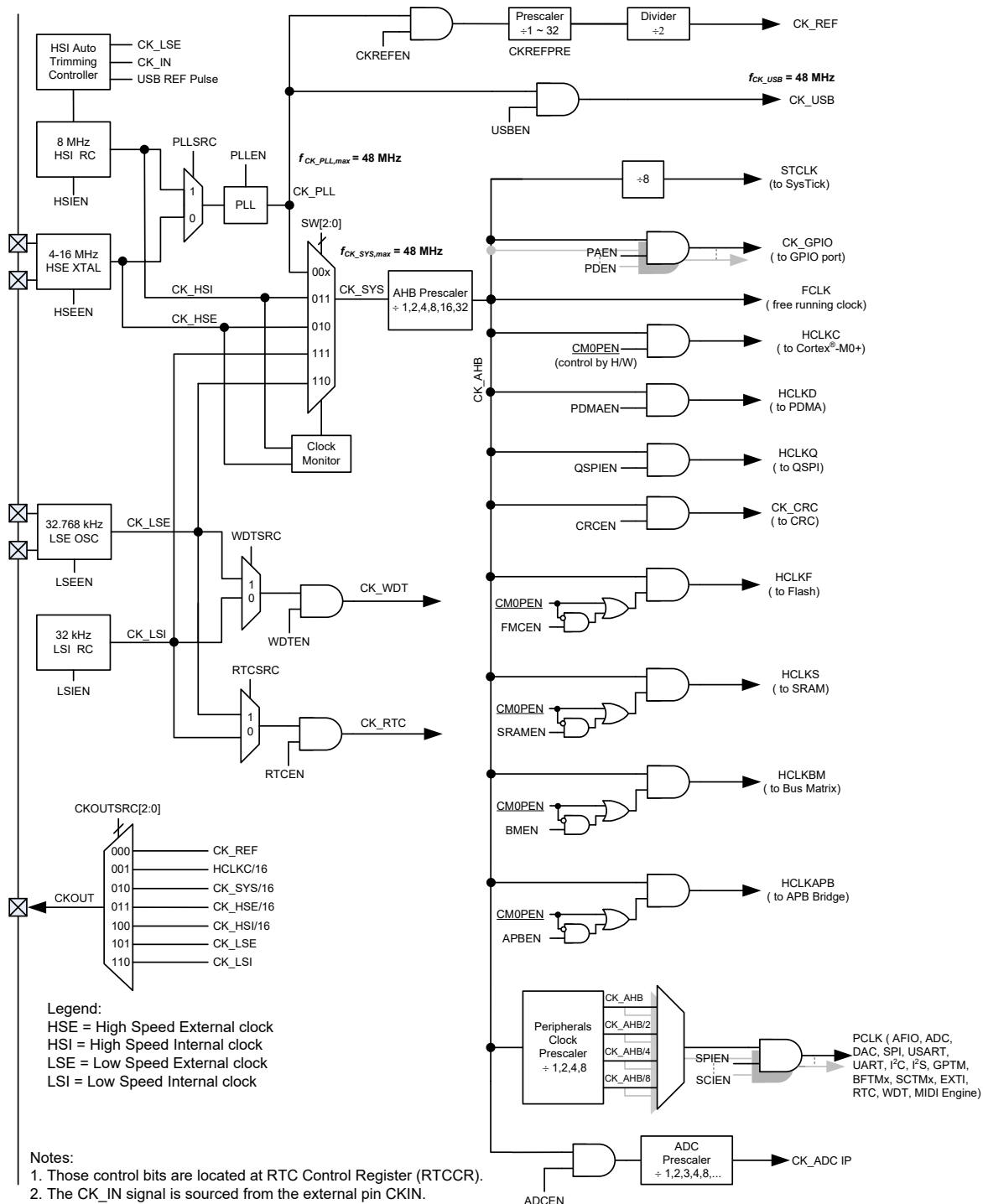
图 3. 时钟结构图
