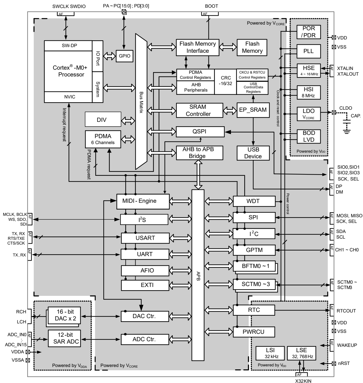
图 1. 方框图
