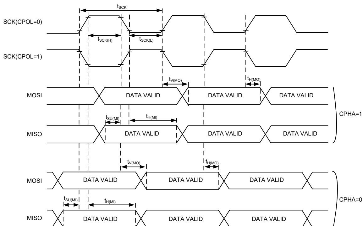
图 12. QSPI 时序图 – QSPI 主机模式 (1-bit 串行模式, DUALEN=0, QUADEN=0)
