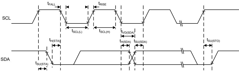
图 9. I²C 时序图
