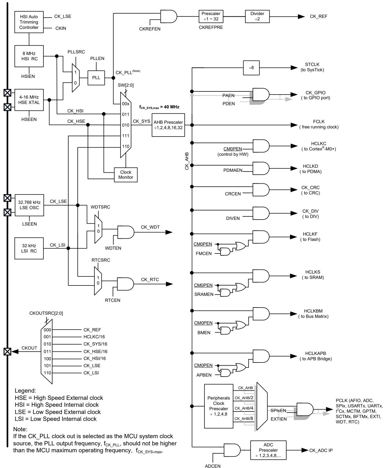
图 3. 时钟结构图
