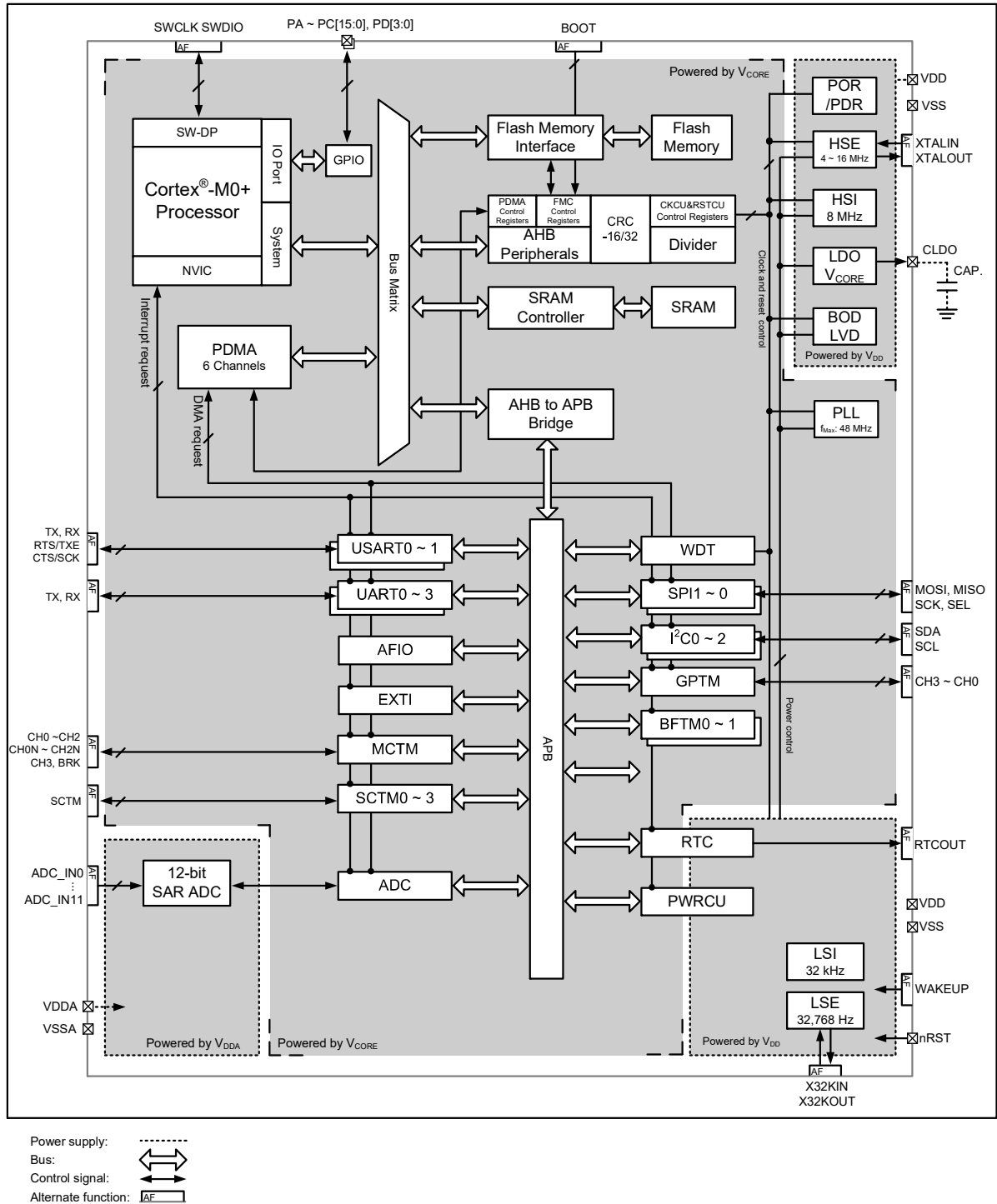
图 1. 方框图
