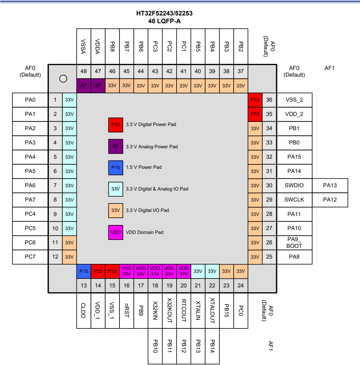
图 6. 48-pin LQFP 引脚图
