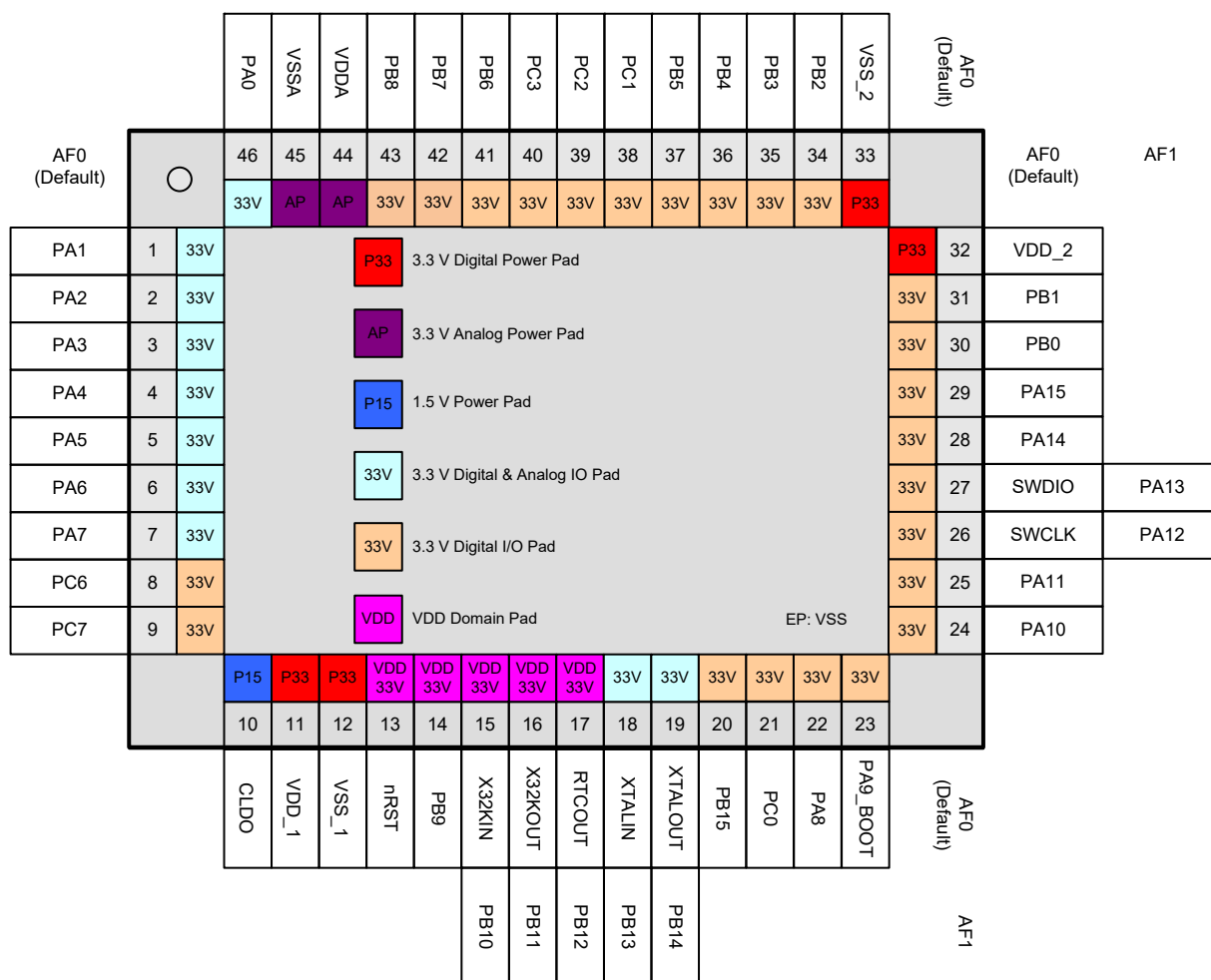
图 5. 46-pin QFN 引脚图
