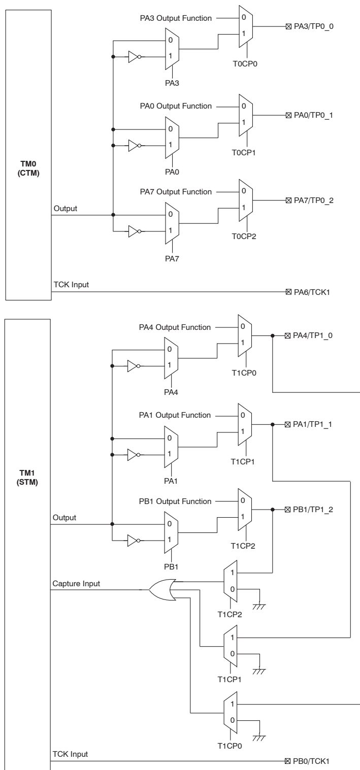
HT66F24D TM0&TM1 功能引脚控制方框图
