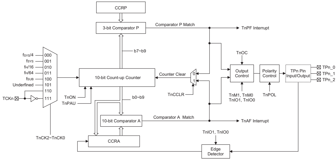
标准型 TM 框图
