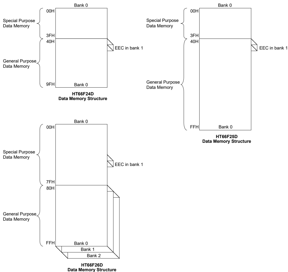
数据存储器结构
