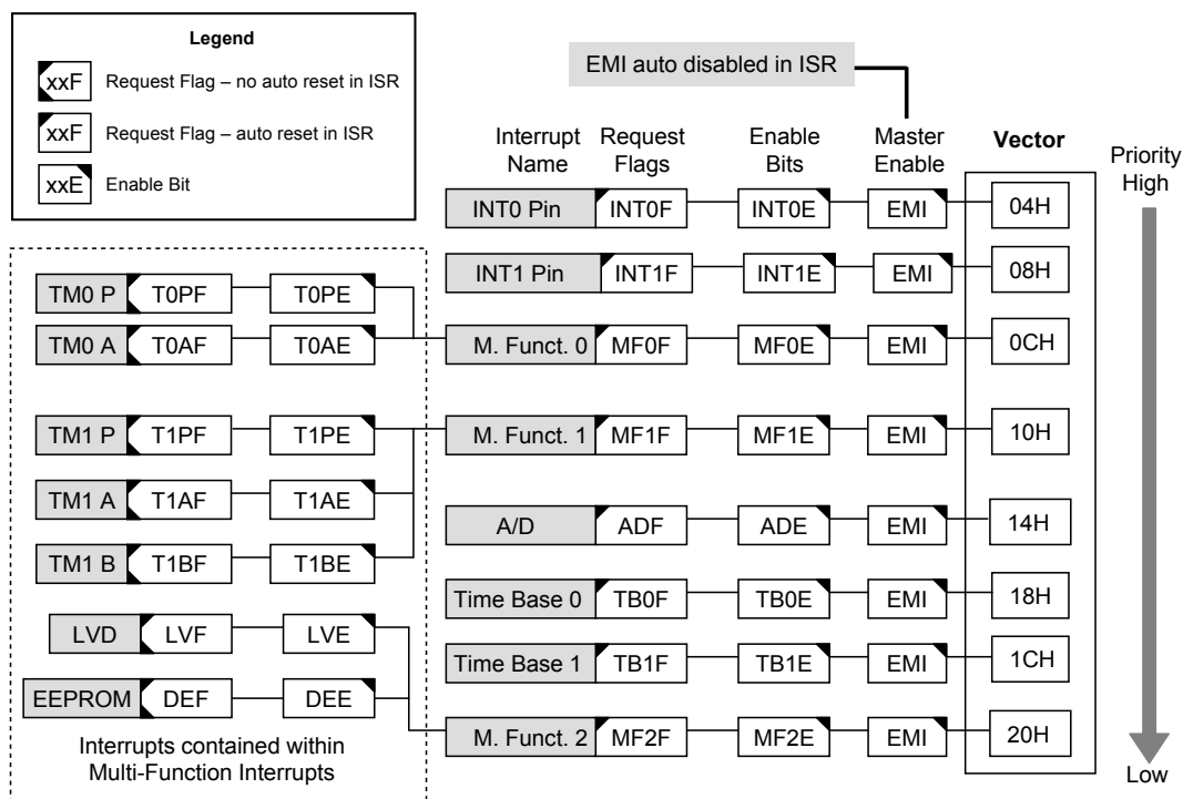
中断结构 – HT66F25D
