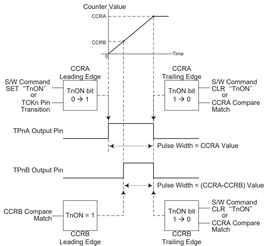
单脉冲产生示意图
