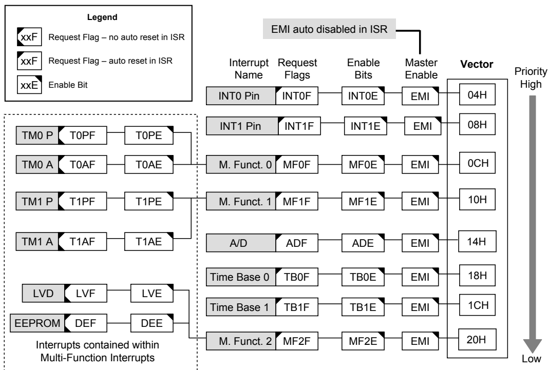
中断结构 – HT66F24D
