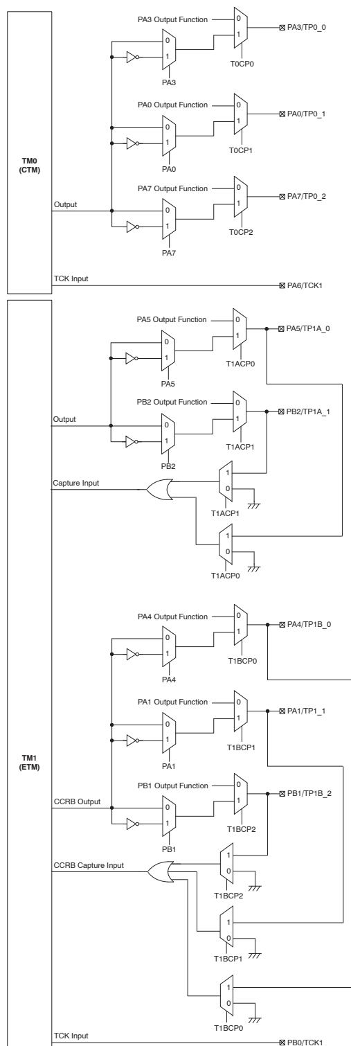
HT66F25D TM0&TM1 功能引脚控制方框图
