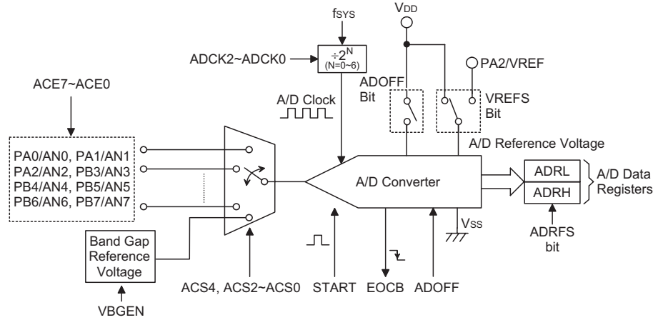
A/D 转换器结构
