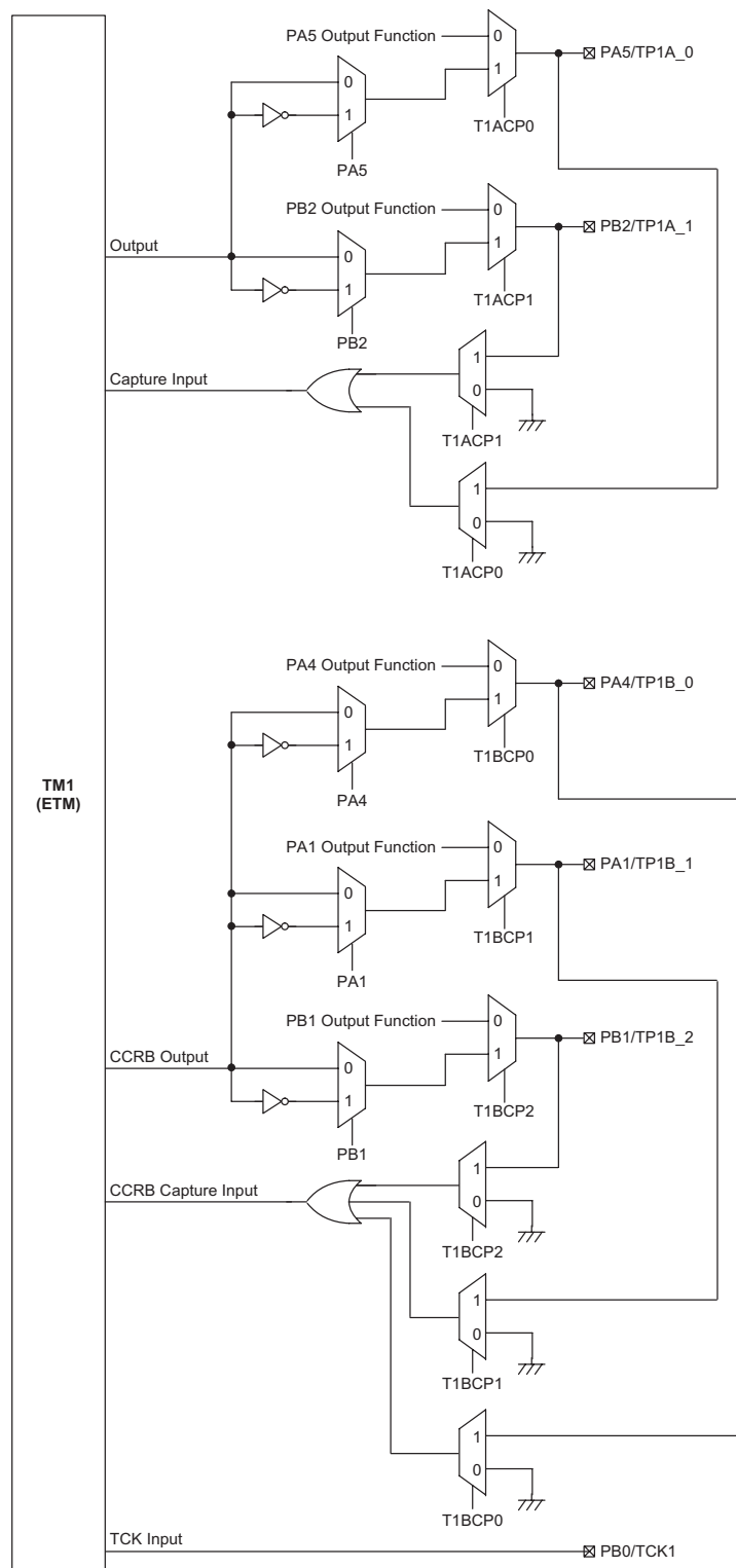
HT66F26D TM 功能引脚控制方框图
