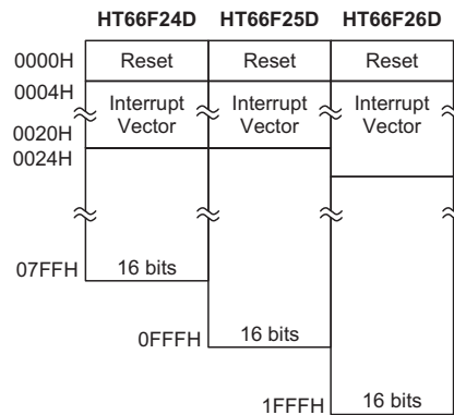
程序存储器结构
