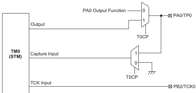
TM0 功能引脚控制方框图 – HT66F318
