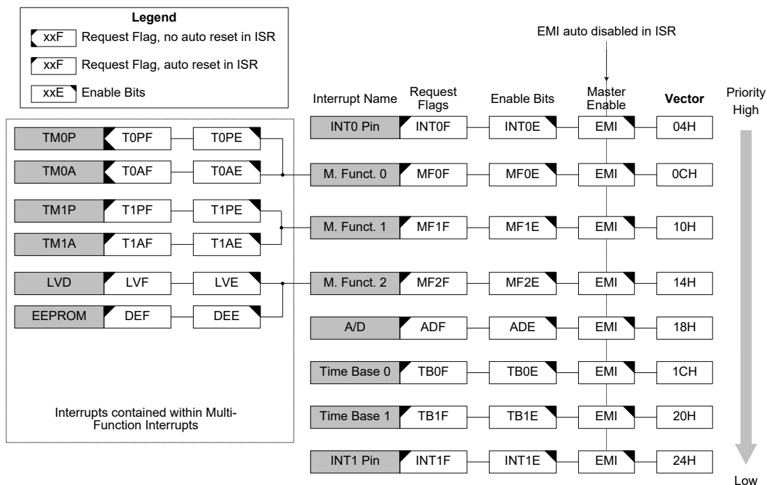
中断结构 – HT66F317
