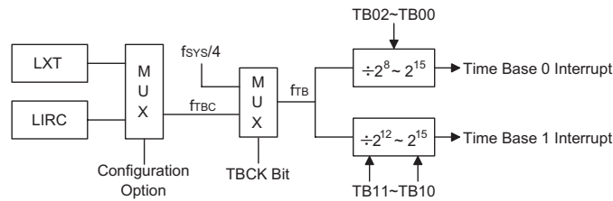
时基中断
