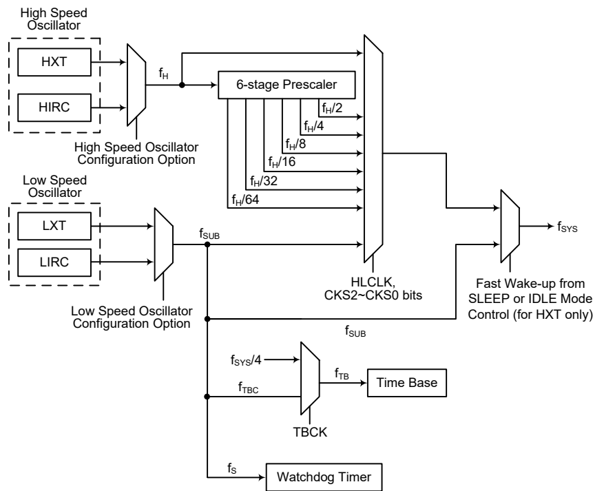
系统时钟选项
