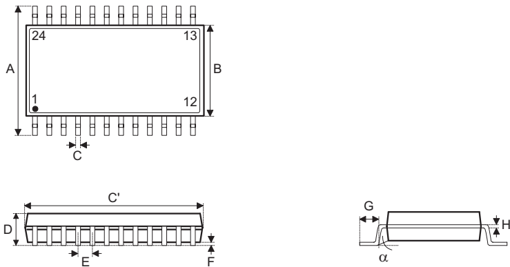
24-pin SSOP (150mil) 外形尺寸
