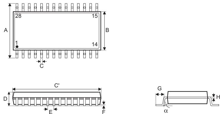
28-pin SOP (300mil) 外形尺寸
