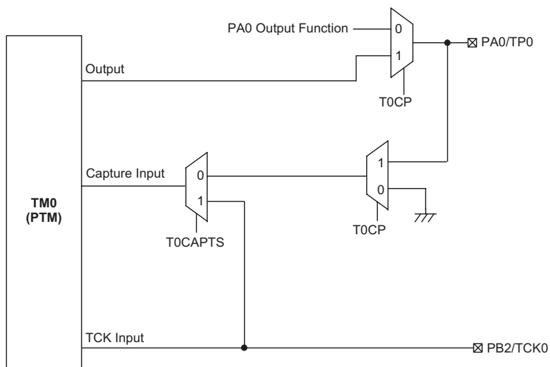
TM0 功能引脚控制方框图 – HT66F317
