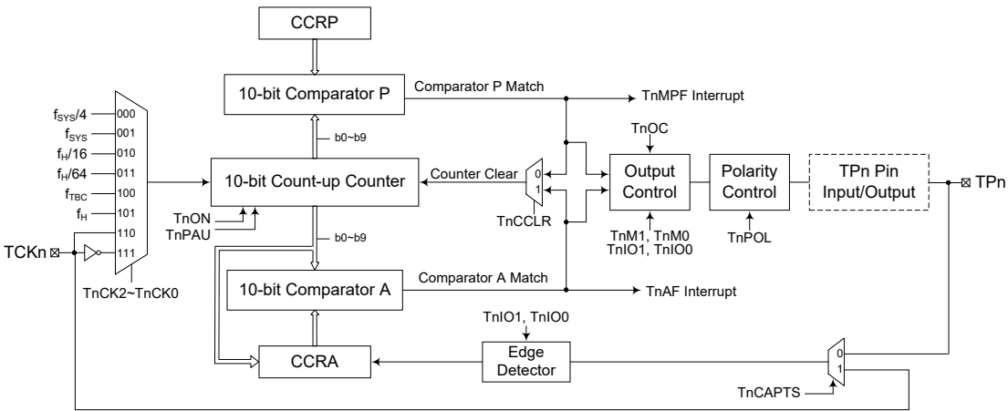
周期型 TM 方框图 (n=0 或 1)
