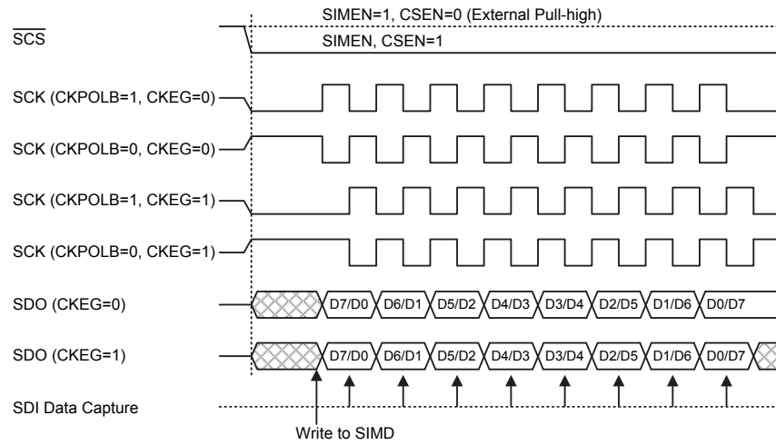
SPI 主机模式时序
