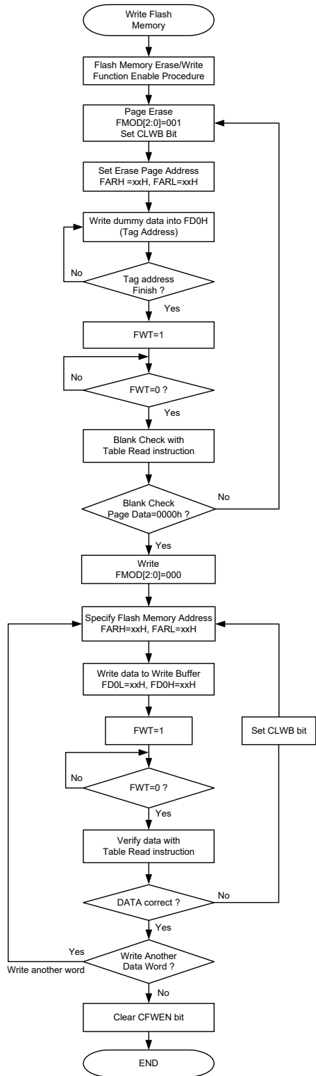
Flash 存储器非连续地址写入程序
