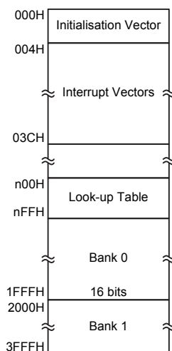
程序存储器结构
