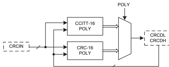
CRC 方框图
