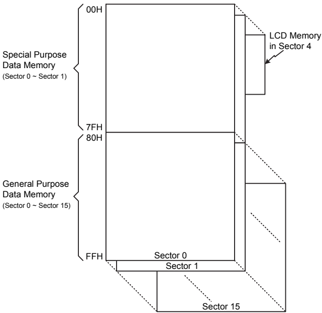
数据存储器结构
