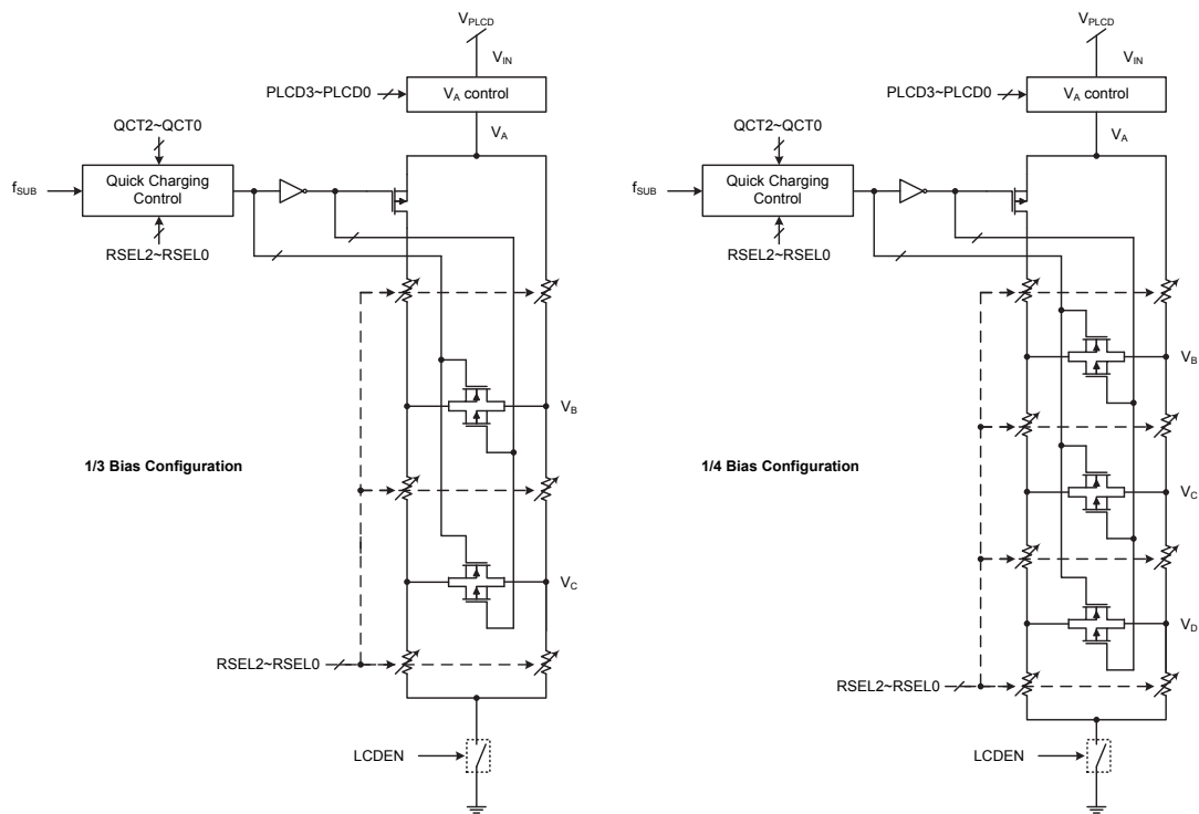
LCD 驱动器输出选项
