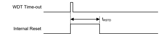
正常运行时看门狗溢出复位时序图
