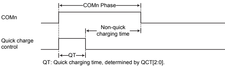
快速充电模式
