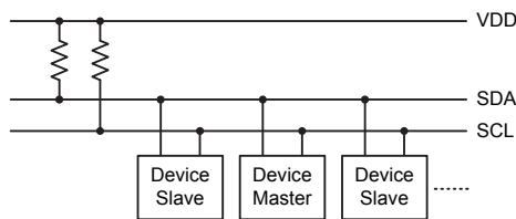
I 2 C 主从总线连接图
