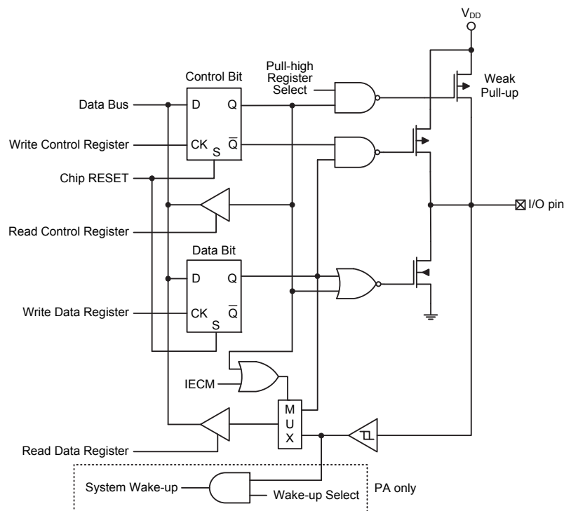
输入 / 输出端口逻辑功能结构
