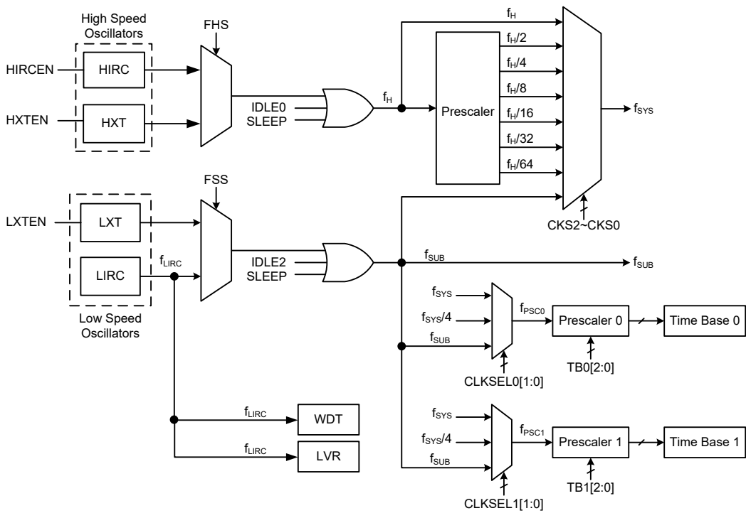
单片机时钟选项
