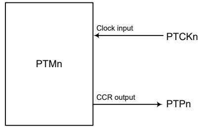
PTM 功能引脚框方图 (n=0~7)
