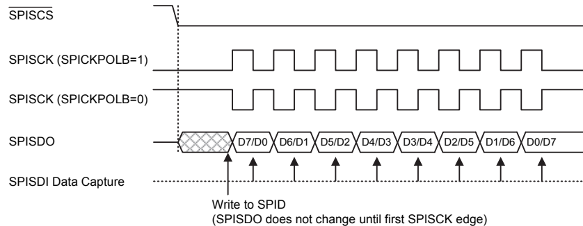
SPI 从机模式时序 – SPICKEG=0
