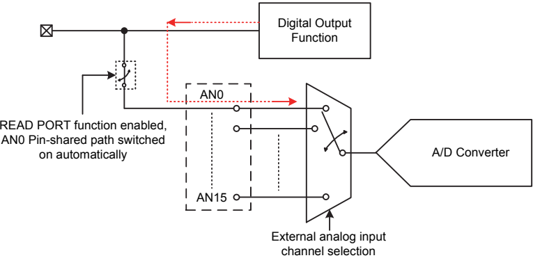
A/D 通道输入路径内部连接
