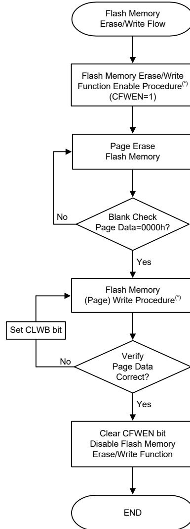
Flash 存储器擦 / 写流程图
