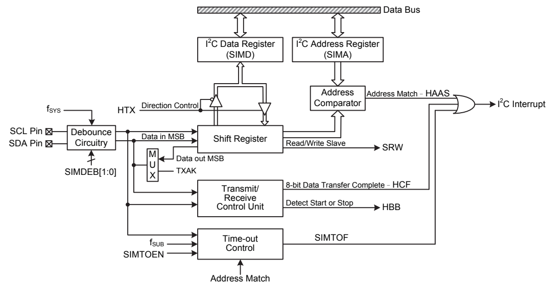
I 2 C 方框图
