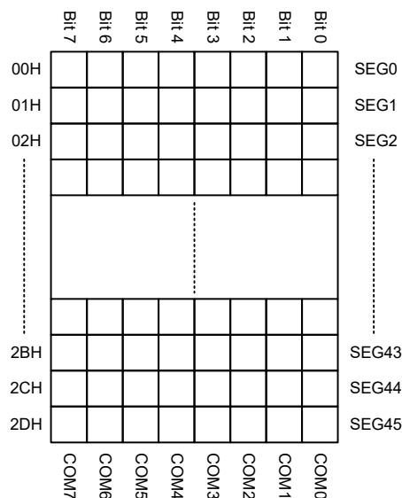
LCD 存储器映射图
