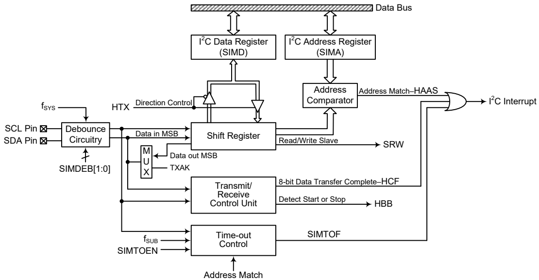
I²C 方框图
