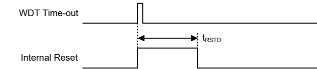
正常运行时看门狗溢出复位时序图
