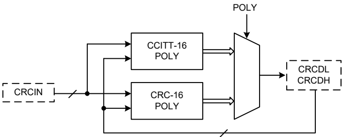
CRC 方框图
