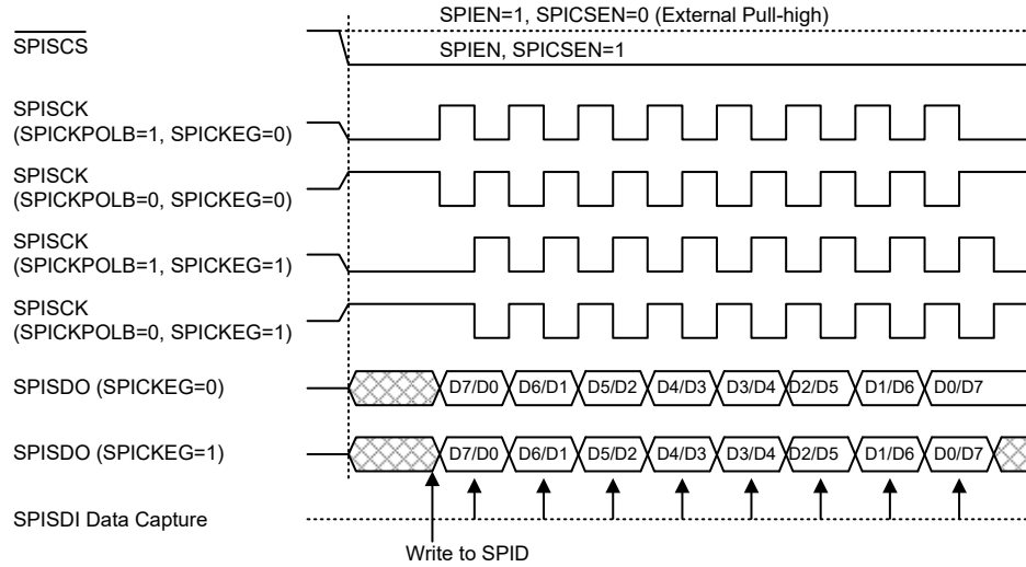
SPI 主机模式时序
