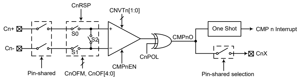
比较器 (n=0~1)
