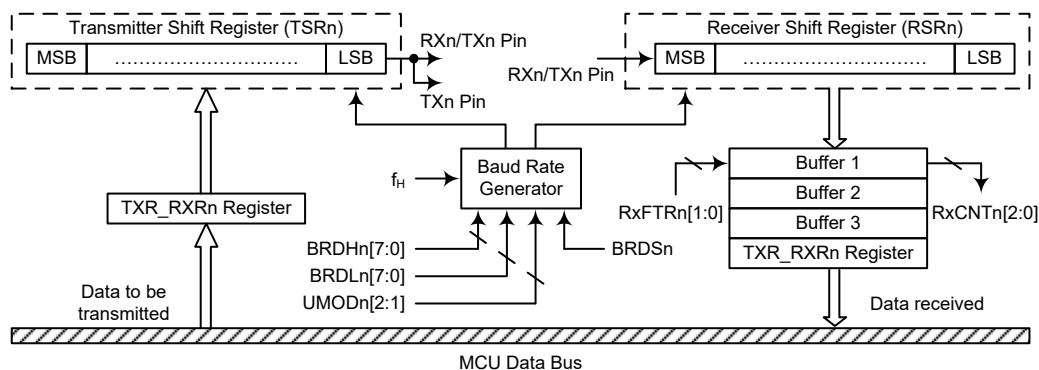
UARTn 数据传输方框图 – SWMn=1 (n=0~2)
