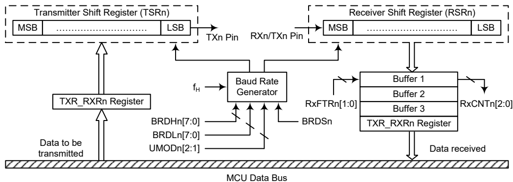
UARTn 数据传输方框图 – SWMn=0 (n=0~2)
