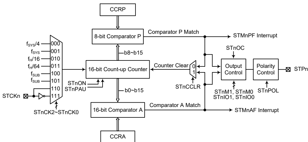
标准型 TM 方框图 (n=0~2)
