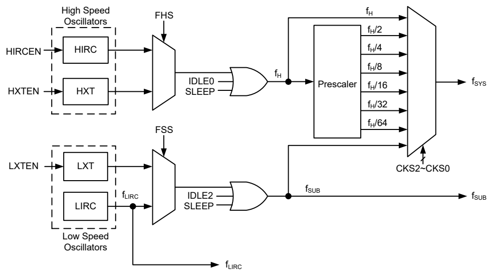
系统时钟配置选项
