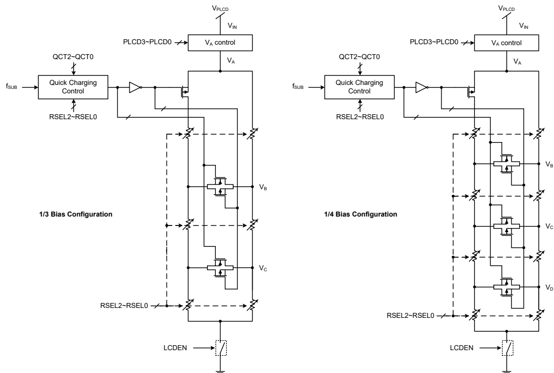
LCD 驱动器输出选项
