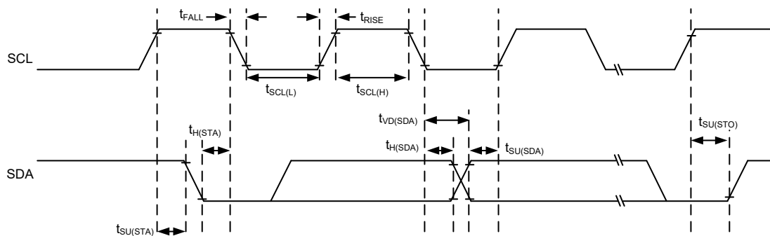
I 2 C 时序图
