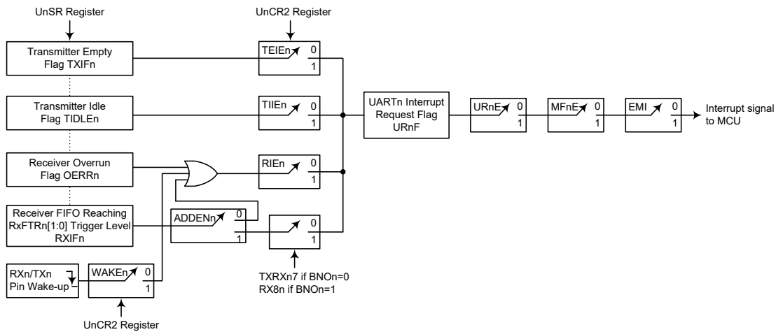
UARTn 中断框图 (n=0~2)
