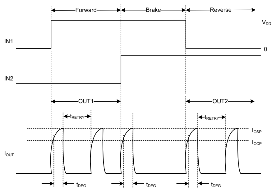
图 5. 重试响应
