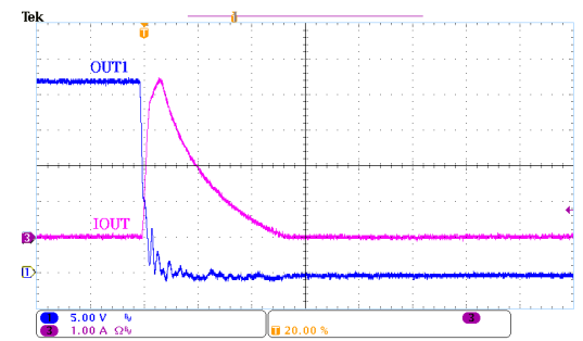
短路保护响应 (放大)
