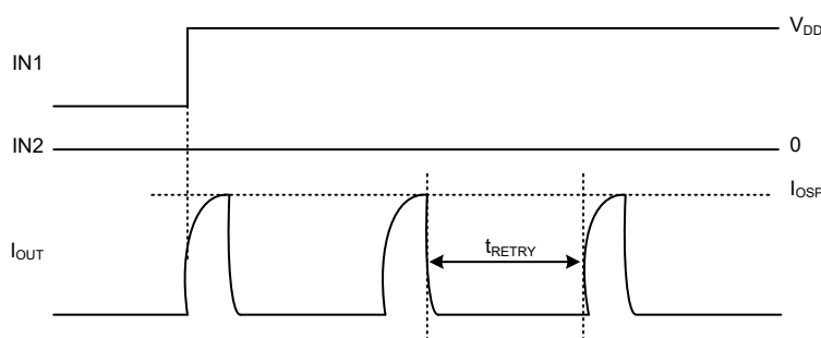
图 4. OSP 响应
