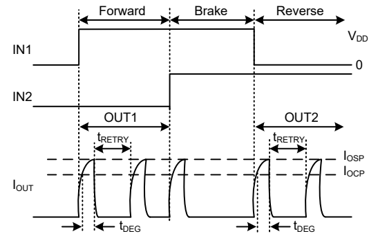
图 6. 重试机制
